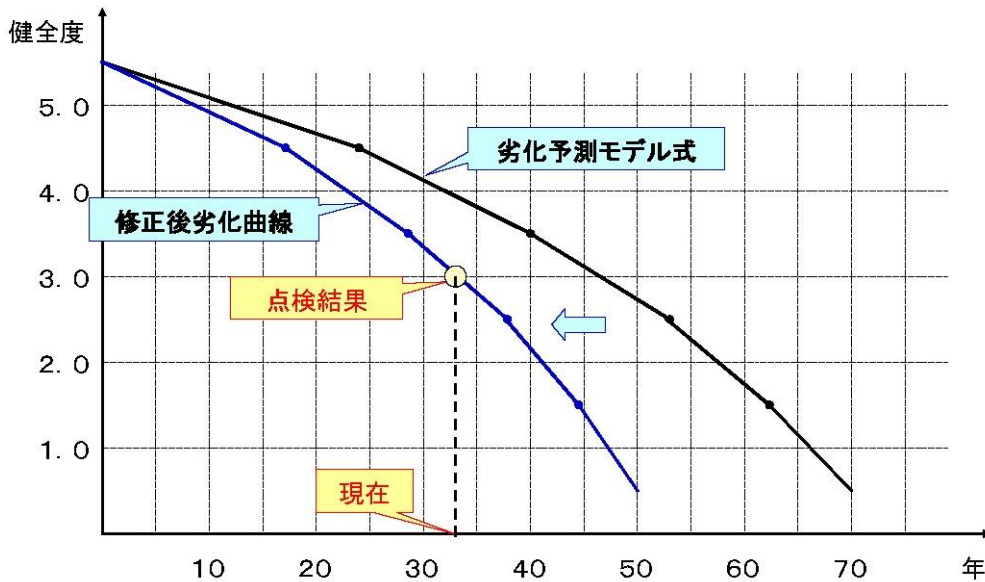
【図-13 劣化予測式の自動修正】
