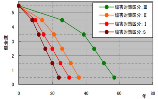
【図-12 劣化予測式の例】 (上部工/R/C/塩害/被覆なし)
