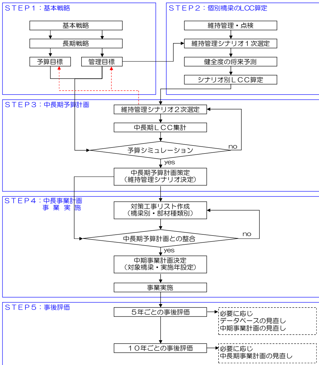
【図-5 BMSを用いたブリッジマネジメントのフロー】
