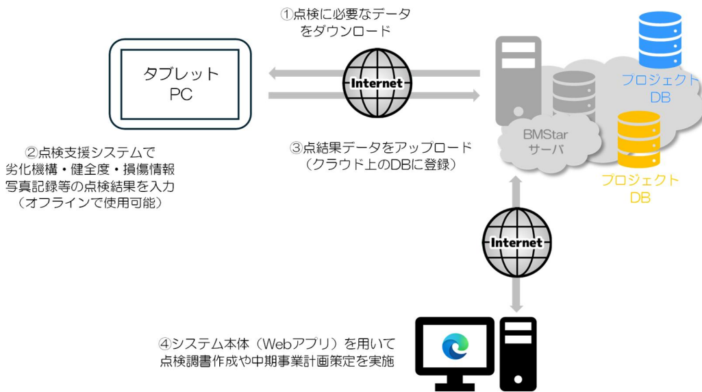
【図-6 BMS 橋梁点検支援システム】
