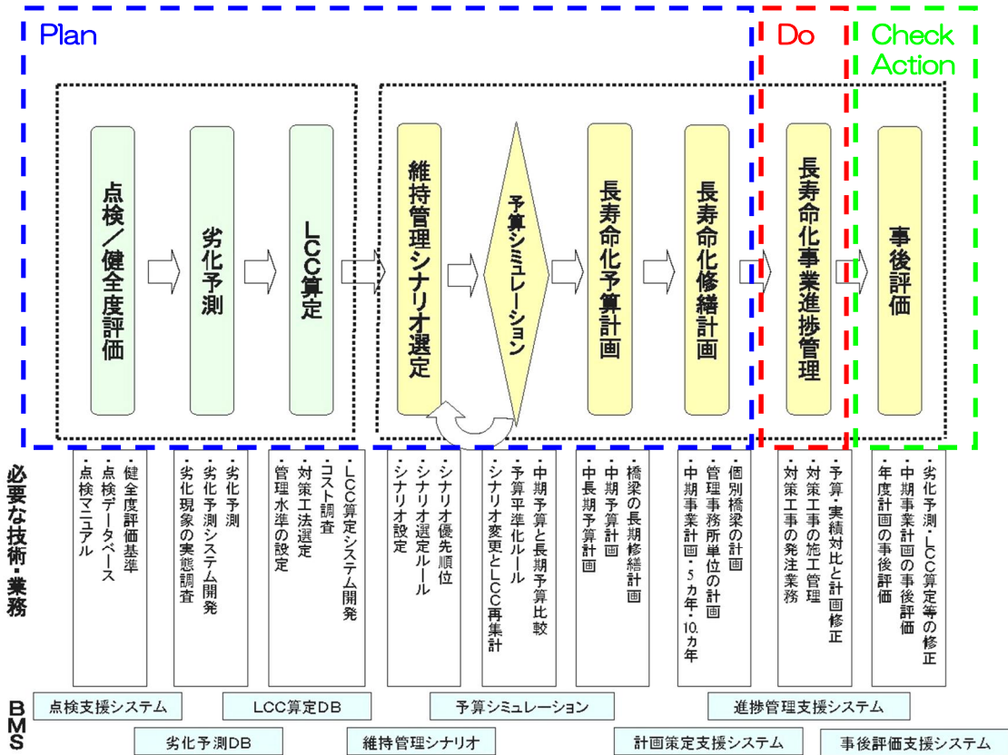
【図-3 橋梁長寿命化修繕計画の基本フロー】
