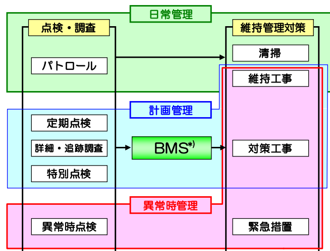
【図-4 維持管理・対策】
