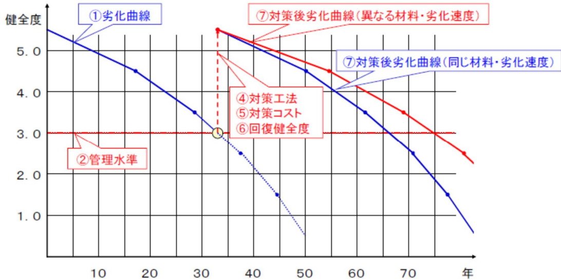
【図-14 LCC算定例・健全度グラフ例】
