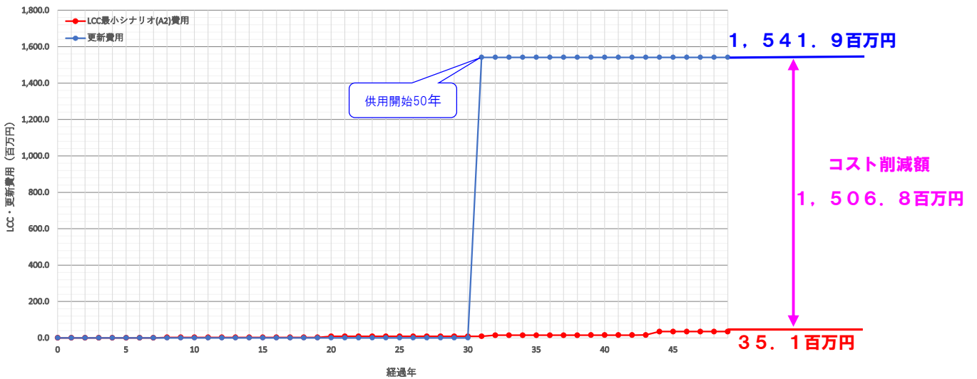
【図-16 コスト削減効果（米沢大橋）】
